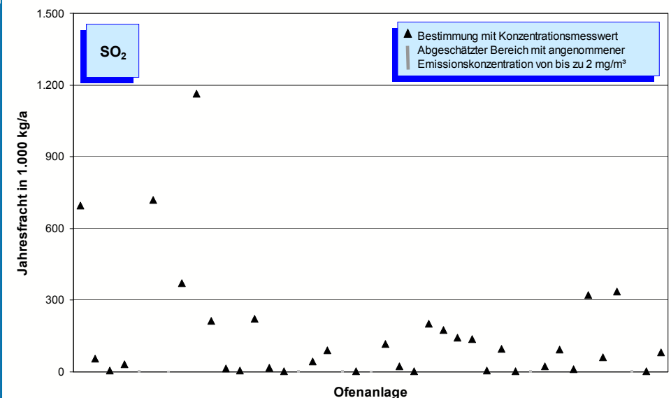
Bild 5-6: SO 2 -Emissionen (Jahresfracht 2010) von 41 Drehofenanlagen. Bei Messungen unterhalb der Nachweisgrenze kann die Fracht nur abgeschätzt werden. Der Bereich möglicher Emissionen ist in diesen Fällen als Linie dargestellt, deren Obergrenze mit einer Konzentration von 2 mg/m 3 berechnet wurde.
