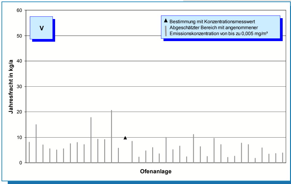
Bild 5-48: Vanadium-Emissionen (Jahresfracht 2010) von 38 Drehofenanlagen.
