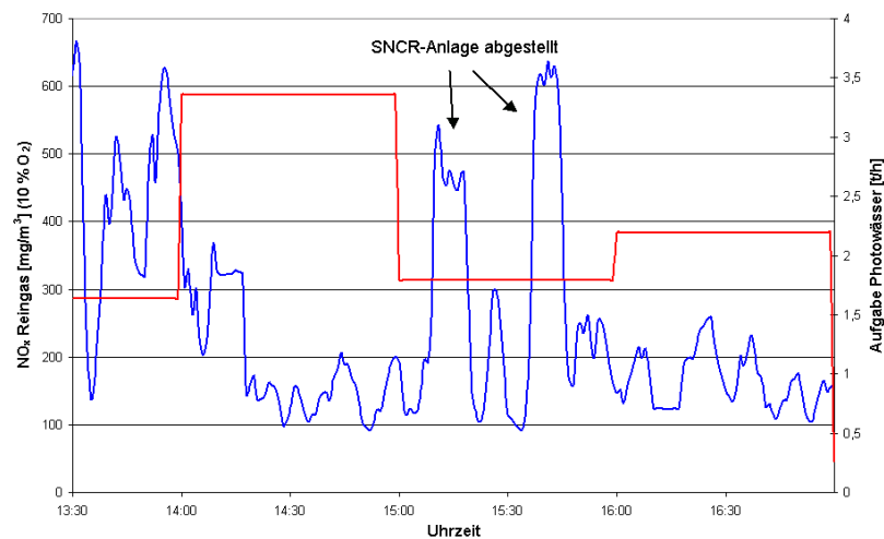
Abb. 1: NO x -Konzentration im Reingas der Drehofenanlage B und Photowasser-Aufgabe (Stundenmittel) bei einem NO x -Zielwert von 200 mg/m 3
