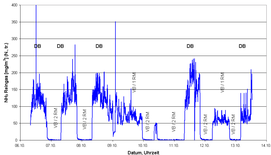
Abb. 2: Kontinuierliche \text{NH}_3 -Messung im Reingaskamin der Ofenanlage C bei einem \text{NO}_x -Zielwert von 200 \text{ mg/m}^3
