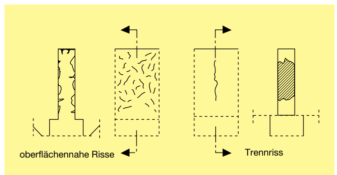
Bild 4: Rissarten
