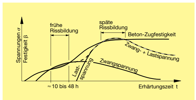
Bild 3: Entwicklung der Betonzugfestigkeit sowie Entstehen von Zwang- und Lastspannungen in Betonbauteilen, nach [2]
