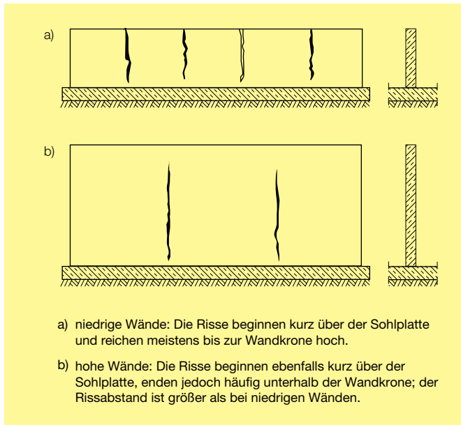
Bild 5: Sichtbare Risse in langen Wänden
