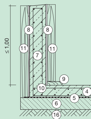
Bild 7: Ortbeton-Bauweise (ohne Arbeitsfuge zwischen Bodenplatte und Wand)
