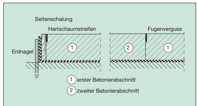
Bild 10: Pressfugenherstellung
