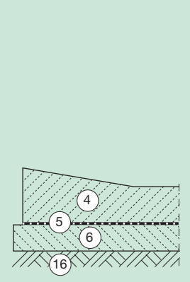
Bild 9: Silierplatte (mit Schweinsrücken)
