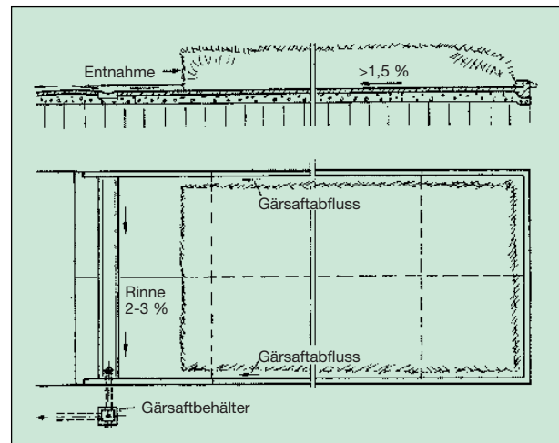
Bild 2: Silierplatte; Grundriss und Schnitt [13]
