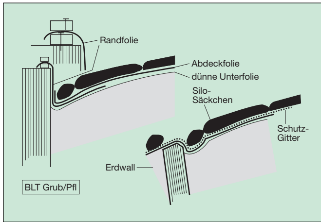
Bild 4: Flachsilo-Abdeckungen; Niederschlagswasser wird vom Futterstock ferngehalten [14]
