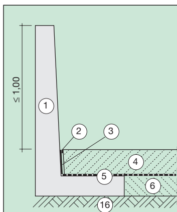
Bild 6: Stahlbetonfertigteil-Bauweise
