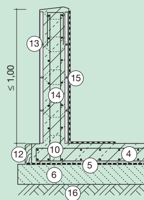
Bild 8: Betonschalungsstein-Bauweise
