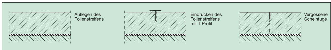
Bild 11: Scheinfugenherstellung
