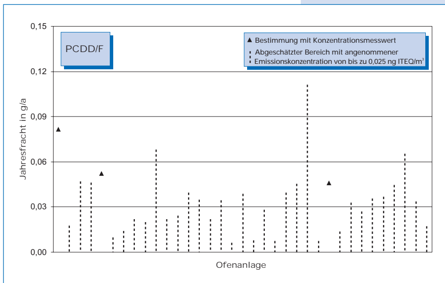
Bild 5-12: Dioxin- und Furan-Emissionen (Jahresfracht 2000) von 35 Drehofenanlagen. Bei Messungen im Bereich der externen Streuung des Verfahrens kann die Fracht nur abgeschätzt werden. Der Bereich möglicher Emissionen ist in diesen Fällen als gestrichelte Linie dargestellt, deren Obergrenze mit einer Konzentration von 0,025 ng ITEQ/m 3 berechnet wurde.
