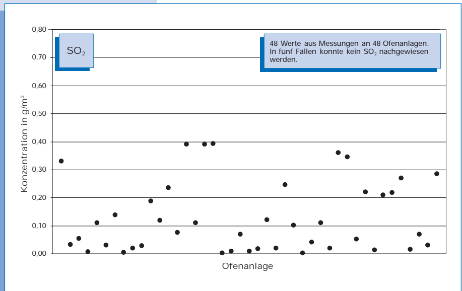
Bild 5-5: Mittelwerte (Jahr 2000) der SO 2 -Konzentration im Reingas von 48 Drehofenanlagen.
