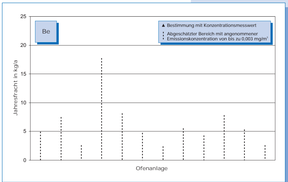
Bild 5-52: Beryllium-Emissionen (Jahresfracht 2000) von zwölf Drehofenanlagen. Bei Messungen unterhalb der Nachweisgrenze kann die Fracht nur abgeschätzt werden. Der Bereich möglicher Emissionen ist in diesen Fällen als gestrichelte Linie dargestellt, deren Obergrenze mit einer Konzentration von 0,003 mg/m 3 berechnet wurde.
