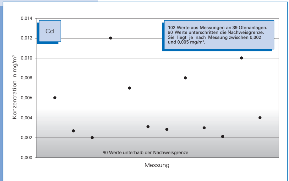
Bild 5-25: Messwerte (Jahr 2000) der Cadmium-Konzentration im Reingas von 39 Drehofenanlagen.
