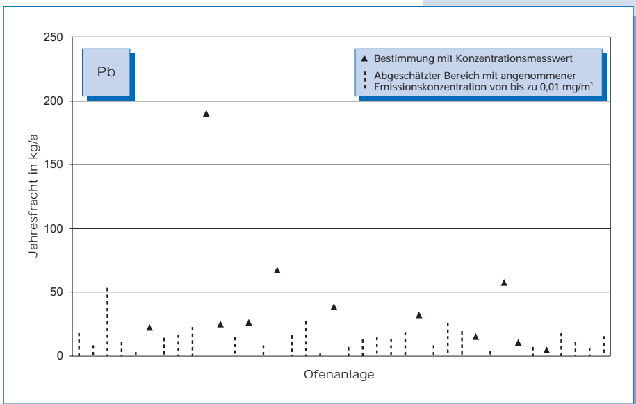
Bild 5-36: Blei-Emissionen (Jahresfracht 2000) von 38 Drehofenanlagen. Bei Messungen unterhalb der Nachweisgrenze kann die Fracht nur abgeschätzt werden. Der Bereich möglicher Emissionen ist in diesen Fällen als gestrichelte Linie dargestellt, deren Obergrenze mit einer Konzentration von 0,01 mg/m 3 berechnet wurde.
