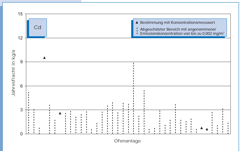
Bild 5-26: Cadmium-Emissionen (Jahresfrachten 2000) von 39 Drehofenanlagen. Bei Messungen unterhalb der Nachweisgrenze kann die Fracht nur abgeschätzt werden. Der Bereich möglicher Emissionen ist in diesen Fällen als gestrichelte Linie dargestellt, deren Obergrenze mit einer Konzentration von 0,002 mg/m 3 berechnet wurde.
