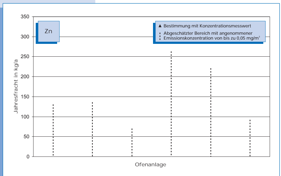
Bild 5-58: Zink-Emissionen (Jahresfracht 2000) von 6 Drehofenanlagen.
