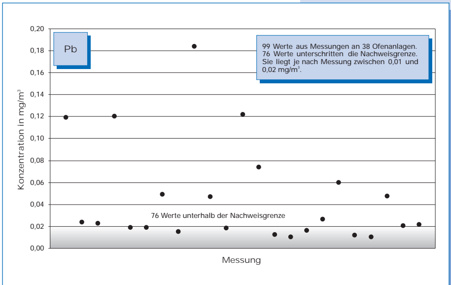
Bild 5-35: Messwerte (Jahr 2000) der Blei-Konzentration im Reingas von 38 Drehofenanlagen.
