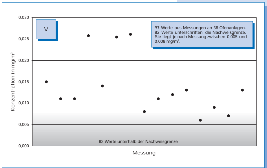
Bild 5-47: Messwerte (Jahr 2000) der Vanadium-Konzentration im Reingas von 38 Drehofenanlagen.
