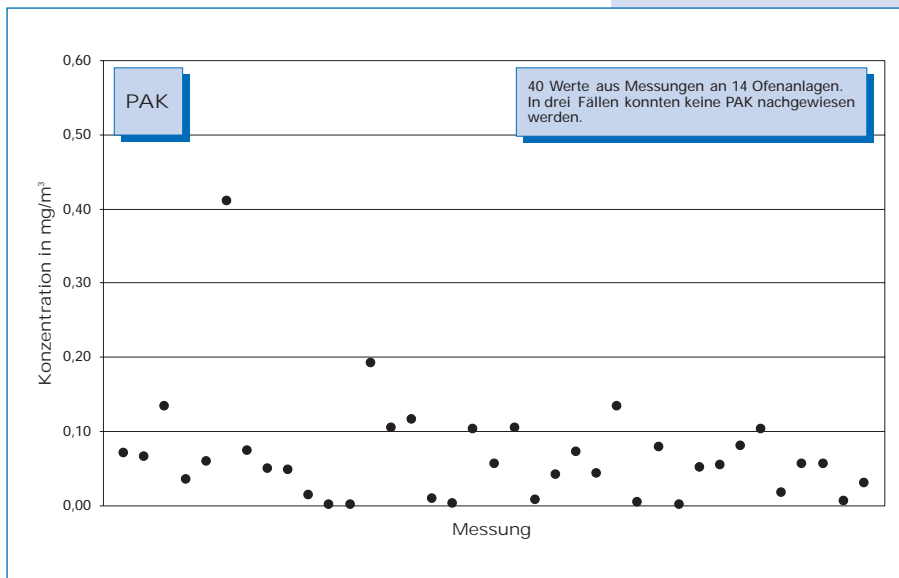
Bild 5-15: Messwerte (Jahr 2000) der Konzentration von polycyclischen aromatischen Kohlenwasserstoffen (PAK nach EPA 610) im Reingas von 14 Drehofenanlagen. In drei Fällen konnten keine PAK nachgewiesen werden. Eine Nachweisgrenze lässt sich aus der Norm nicht ableiten. Bei den derzeit eingesetzten Messverfahren sind gemessene Emissionskonzentrationen unterhalb von 0,01 \text{ mg/m}^3 nicht abgesichert.
