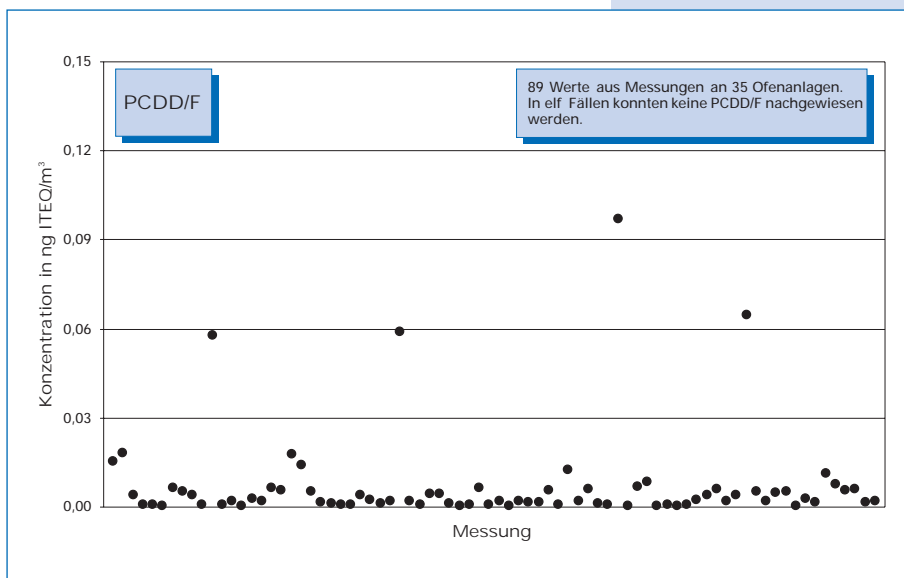
Bild 5-11: Messwerte (Jahr 2000) der Konzentration von Dioxinen und Furanen (PCDD/F) im Reingas von 35 Drehofenanlagen. In elf Fällen konnten keine PCDD/F nachgewiesen werden. Anmerkung: Aus der Norm lässt sich keine Nachweisgrenze ableiten. Für die Beurteilung der Messergebnisse kann die externe Streuung des Verfahrens (Vergleich verschiedener Laboratorien) herangezogen werden. Sie beträgt gemäß DIN EN 1948 \pm 0,05 ng ITEQ/m 3 . (ITEQ: Internationales Toxizitätsäquivalent)
