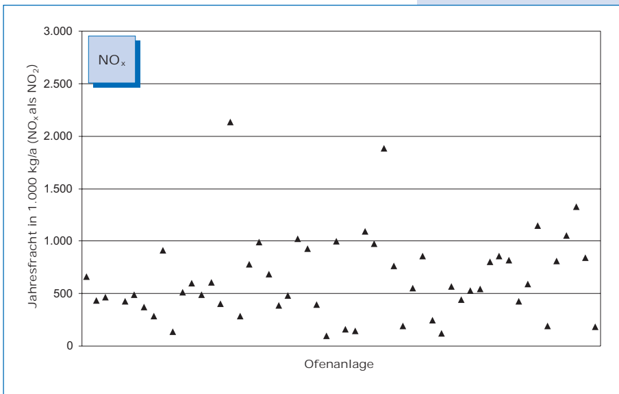
Bild 5-4: NO x -Emissionen (Jahresfracht 2000) von 54 Drehofenanlagen.
