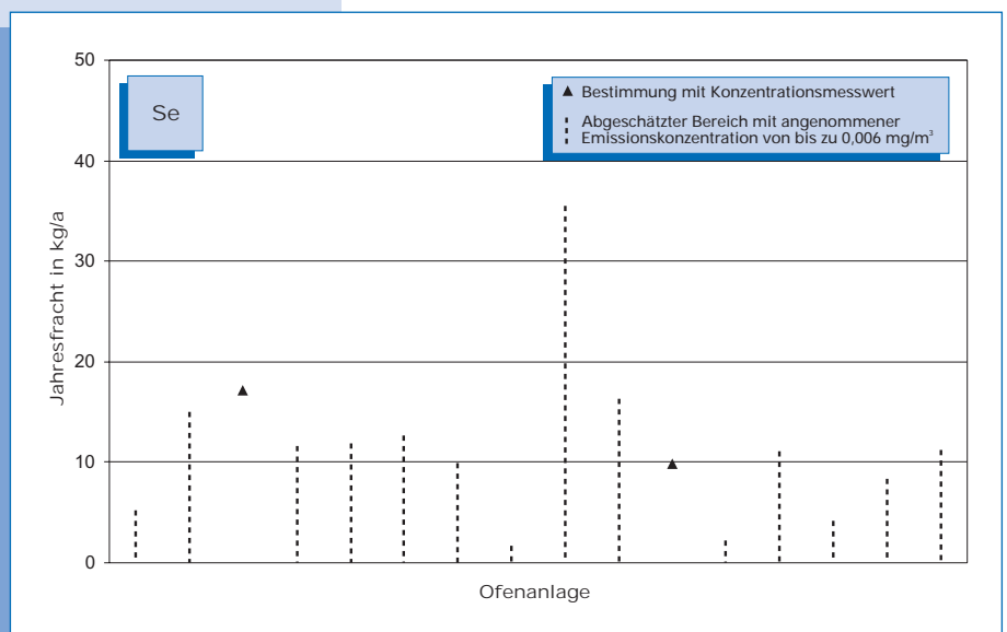
Bild 5-54: Selen-Emissionen (Jahresfracht 2000) von 16 Drehofenanlagen. Bei Messungen unterhalb der Nachweisgrenze kann die Fracht nur abgeschätzt werden. Der Bereich möglicher Emissionen ist in diesen Fällen als gestrichelte Linie dargestellt, deren Obergrenze mit einer Konzentration von 0,006 mg/m 3 berechnet wurde.
