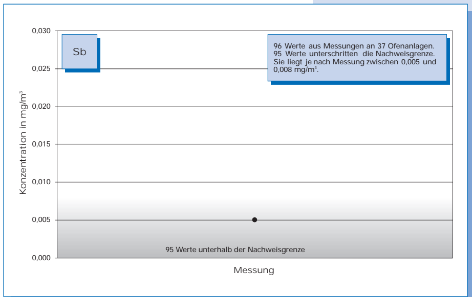
Bild 5-31: Messwerte (Jahr 2000) der Antimon-Konzentration im Reingas von 37 Drehofenanlagen.
