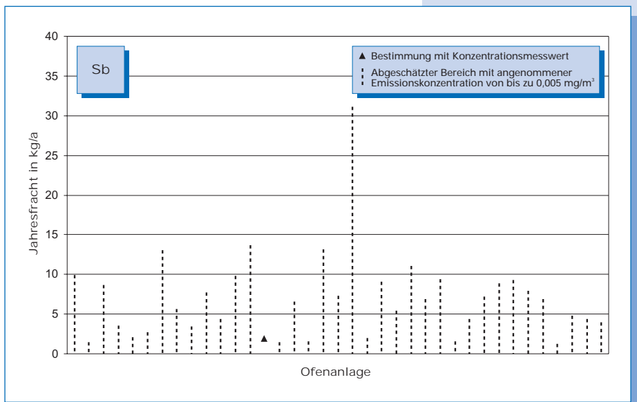
Bild 5-32: Antimon-Emissionen (Jahresfrachten 2000) von 37 Drehofenanlagen. Bei Messungen unterhalb der Nachweisgrenze kann die Fracht nur abgeschätzt werden. Der Bereich möglicher Emissionen ist in diesen Fällen als gestrichelte Linie dargestellt, deren Obergrenze mit einer Konzentration von 0,005 mg/m 3 berechnet wurde.
