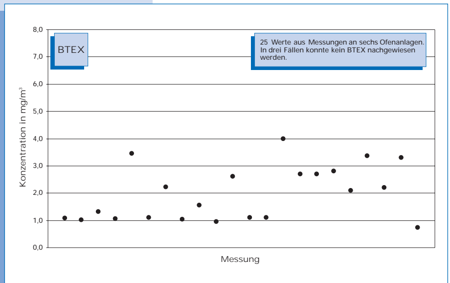
Bild 5-17: Messwerte (Jahr 2000) der Konzentration von BTEX im Reingas von sechs Drehofenanlagen. In drei Fällen konnte kein BTEX nachgewiesen werden.
