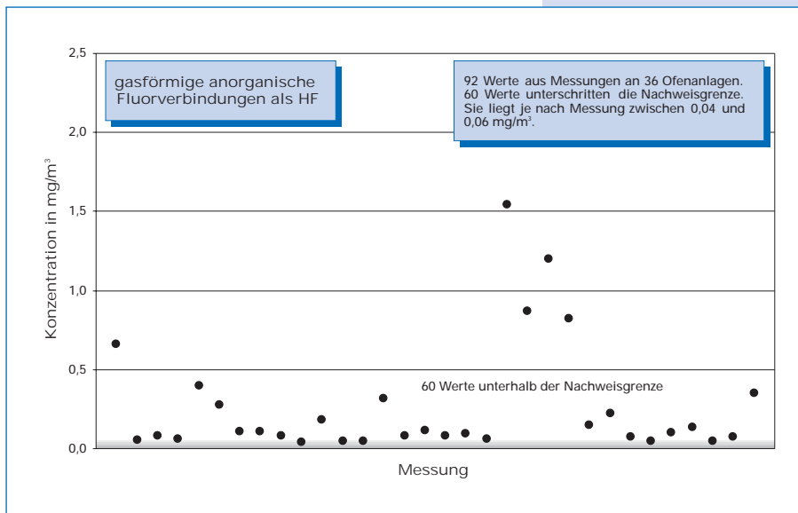
Bild 5-23: Messwerte (Jahr 2000) der Konzentration gasförmiger anorganischer Fluorverbindungen, berechnet als HF, im Reingas von 36 Drehofenanlagen.
