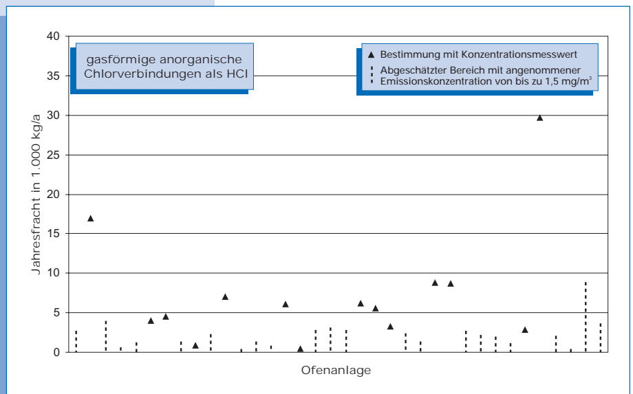
Bild 5-22: HCl-Emissionen (Jahresfracht 2000) von 36 Drehofenanlagen.
