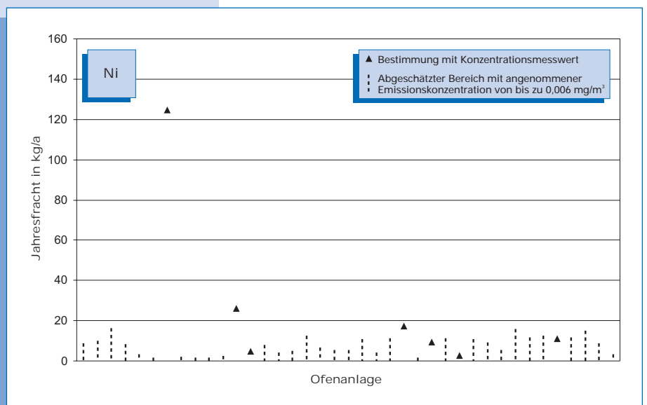
Bild 5-46: Nickel-Emissionen (Jahresfracht 2000) von 39 Drehofenanlagen. Bei Messungen unterhalb der Nachweisgrenze kann die Fracht nur abgeschätzt werden. Der Bereich möglicher Emissionen ist in diesen Fällen als gestrichelte Linie dargestellt, deren Obergrenze mit einer Konzentration von 0,006 mg/m 3 berechnet wurde.
