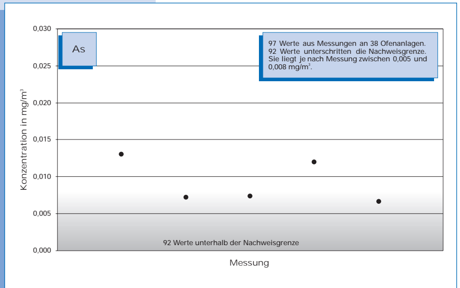
Bild 5-33: Messwerte (Jahr 2000) der Arsen-Konzentration im Reingas von 38 Drehofenanlagen.
