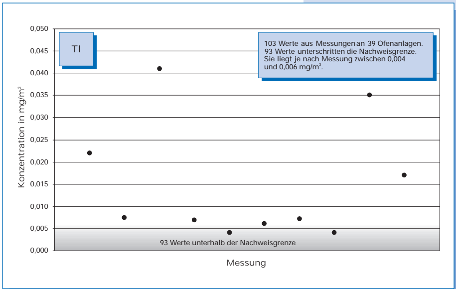
Bild 5-27: Messwerte (Jahr 2000) der Thallium-Konzentration im Reingas von 39 Drehofenanlagen.
