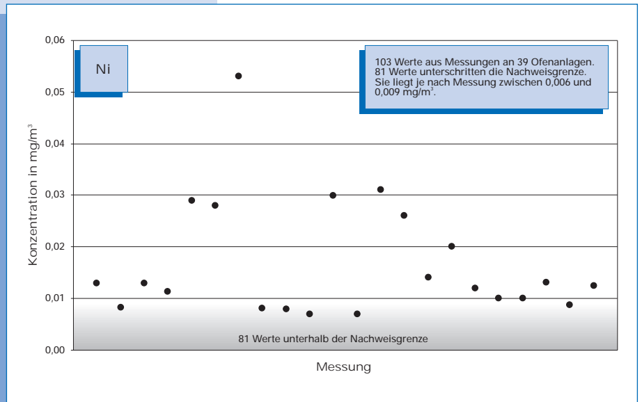
Bild 5-45: Messwerte (Jahr 2000) der Nickel-Konzentration im Reingas von 39 Drehofenanlagen.
