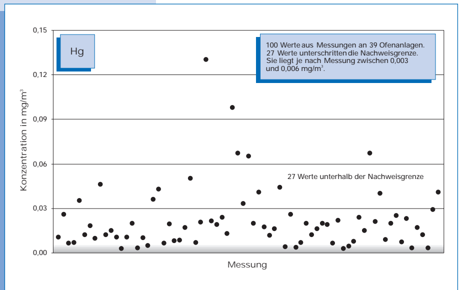
Bild 5-29: Messwerte (Jahr 2000) der Quecksilber-Konzentration im Reingas von 39 Drehofenanlagen.
