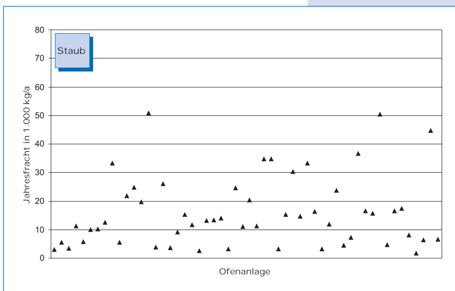
Bild 5-2: Staub-Emissionen (Jahresfracht 2000) von 54 Drehofenanlagen.
