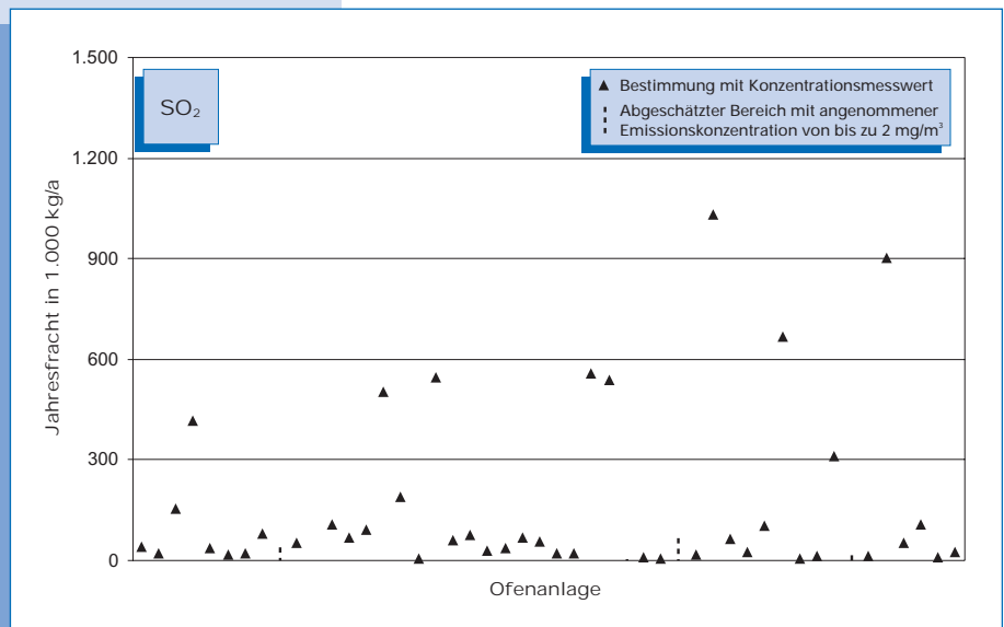
Bild 5-6: SO 2 -Emissionen (Jahresfracht 2000) von 48 Drehofenanlagen.
