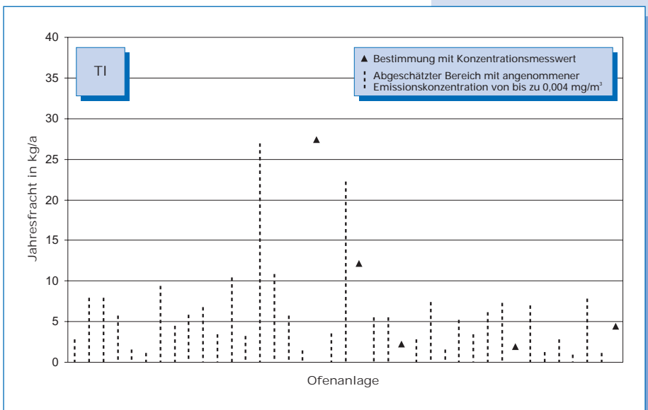
Bild 5-28: Thallium-Emissionen (Jahresfracht 2000) von 39 Drehofenanlagen. Bei Messungen unterhalb der Nachweisgrenze kann die Fracht nur abgeschätzt werden. Der Bereich möglicher Emissionen ist in diesen Fällen als gestrichelte Linie dargestellt, deren Obergrenze mit einer Konzentration von 0,004 mg/m 3 berechnet wurde.
