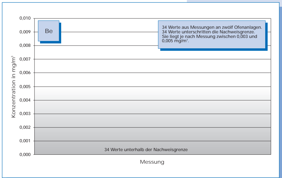
Bild 5-51: Messwerte (Jahr 2000) der Beryllium-Konzentration im Reingas von zwölf Drehofenanlagen.
