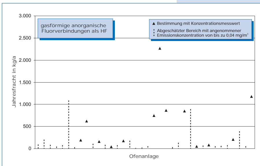
Bild 5-24: HF-Emissionen (Jahresfracht 2000) von 36 Drehofenanlagen.
