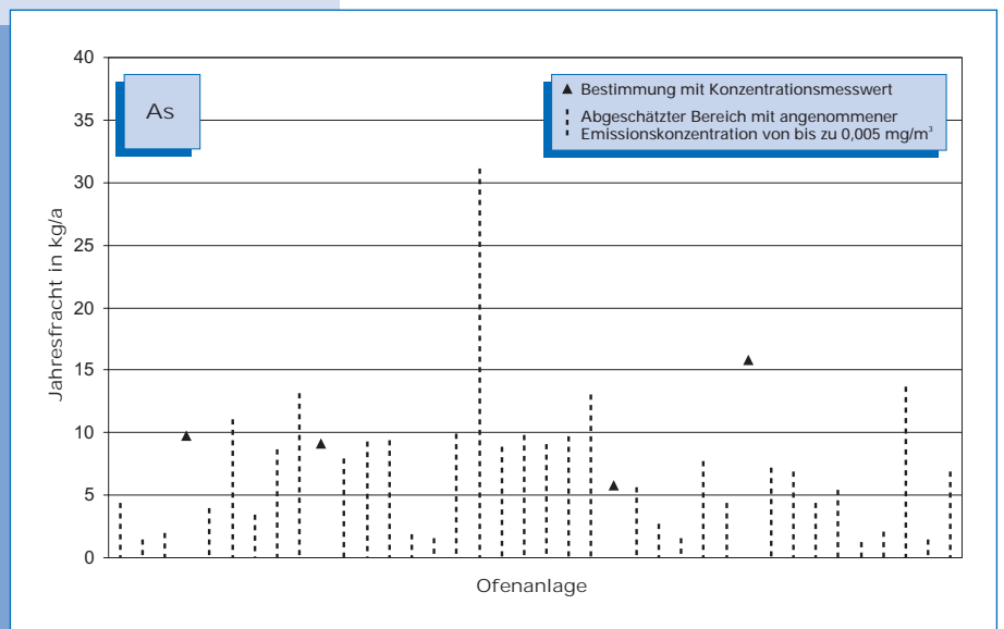
Bild 5-34: Arsen-Emissionen (Jahresfracht 2000) von 38 Drehofenanlagen. Bei Messungen unterhalb der Nachweisgrenze kann die Fracht nur abgeschätzt werden. Der Bereich möglicher Emissionen ist in diesen Fällen als gestrichelte Linie dargestellt, deren Obergrenze mit einer Konzentration von 0,005 mg/m 3 berechnet wurde.
