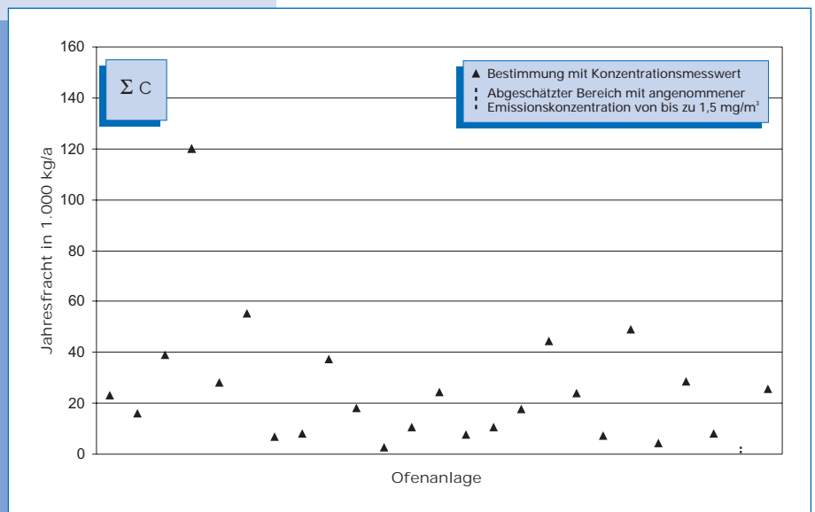
Bild 5-10: Emissionen von organischem Gesamtkohlenstoff (Jahresfracht 2000) von 25 Drehofenanlagen. Bei Messungen unterhalb der Nachweisgrenze kann die Fracht nur abgeschätzt werden. Der Bereich möglicher Emissionen ist in diesen Fällen als gestrichelte Linie dargestellt, deren Obergrenze mit einer Konzentration von 1,5 mg/m 3 berechnet wurde.
