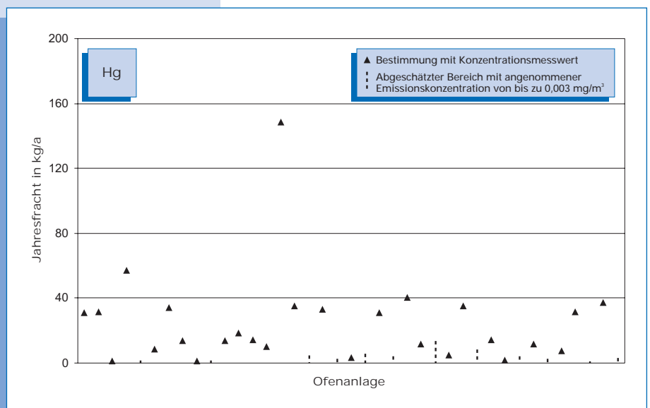
Bild 5-30: Quecksilber-Emissionen (Jahresfracht 2000) von 39 Drehofenanlagen. Bei Messungen unterhalb der Nachweisgrenze kann die Fracht nur abgeschätzt werden. Der Bereich möglicher Emissionen ist in diesen Fällen als gestrichelte Linie dargestellt, deren Obergrenze mit einer Konzentration von 0,003 \text{ mg/m}^3 berechnet wurde.
