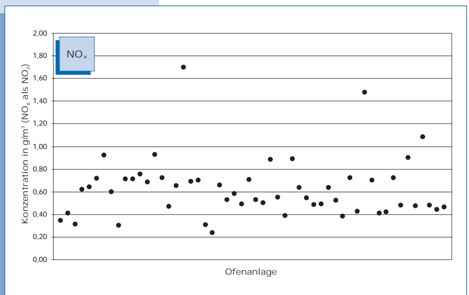
Bild 5-3: Mittelwerte (Jahr 2000) der NO x -Konzentration im Reingas von 54 Drehofenanlagen. Anmerkung: Im Jahr 2000 überstiegen die Emissionen mehrerer Anlagen die heute in der TA Luft für Zementwerke vorgesehenen Emissionswerte. Die Betriebsgenehmigungen für diese Werke beruhen noch auf höheren NO x -Grenzwerten. Einige dieser Anlagen sind bzw. werden in den nächsten Jahren stillgelegt, weitere werden mit einer Anlage zur NO x -Minderung nachgerüstet.
