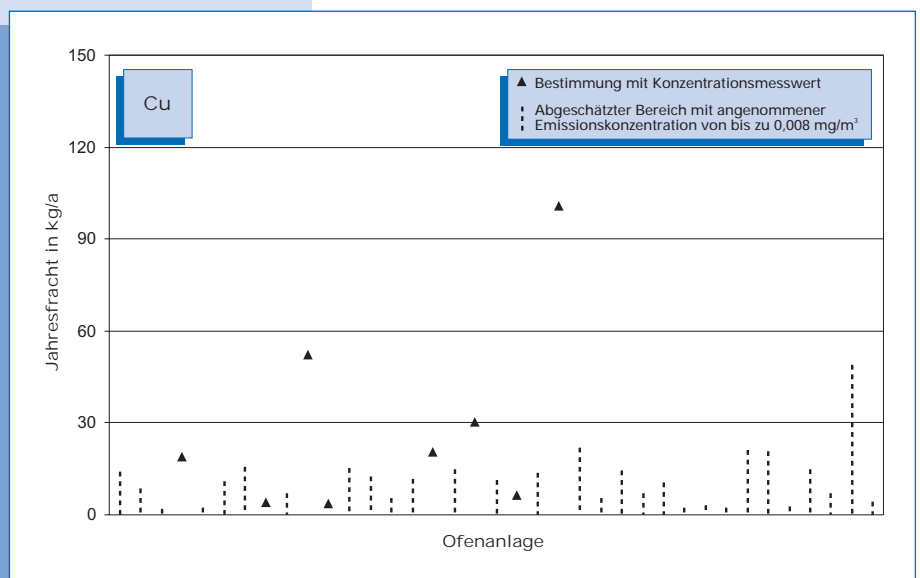
Bild 5-42: Kupfer-Emissionen (Jahresfracht 2000) von 37 Drehofenanlagen. Bei Messungen unterhalb der Nachweisgrenze kann die Fracht nur abgeschätzt werden. Der Bereich möglicher Emissionen ist in diesen Fällen als gestrichelte Linie dargestellt, deren Obergrenze mit einer Konzentration von 0,008 mg/m 3 berechnet wurde.
