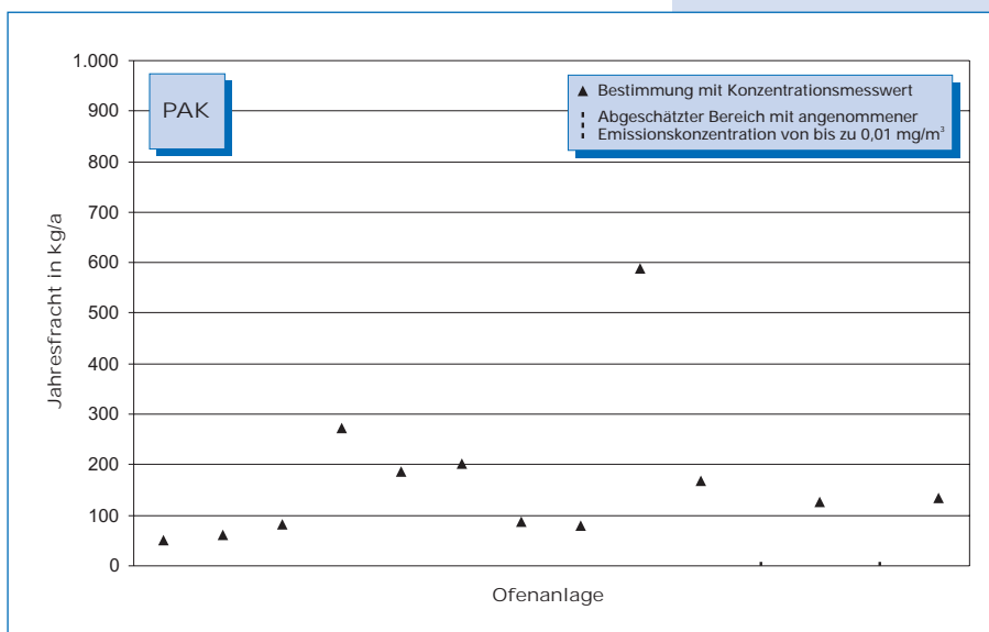
Bild 5-16: PAK-Emissionen (Jahresfracht 2000) von 14 Drehofenanlagen. Bei nicht abgesicherten Messungen kann die Fracht nur abgeschätzt werden. Der Bereich möglicher Emissionen ist in diesen Fällen als gestrichelte Linie dargestellt, deren Obergrenze mit einer Konzentration von 0,01 \text{ mg/m}^3 berechnet wurde.
