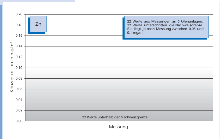
Bild 5-57: Messwerte (Jahr 2000) der Zink-Konzentration im Reingas von 6 Drehofenanlagen.
