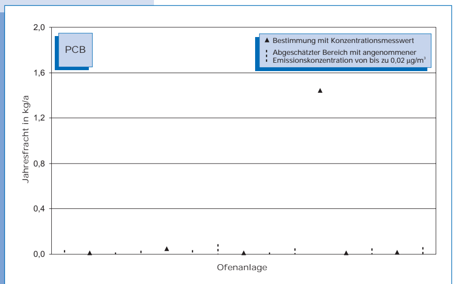
Bild 5-14: PCB-Emissionen (Jahresfracht 2000) von 15 Drehofenanlagen. Bei nicht abgesicherten Messungen kann die Fracht nur abgeschätzt werden. Der Bereich möglicher Emissionen ist in diesen Fällen als gestrichelte Linie dargestellt, deren Obergrenze mit einer Konzentration von 0,02 \mu\text{g}/\text{m}^3 berechnet wurde.
