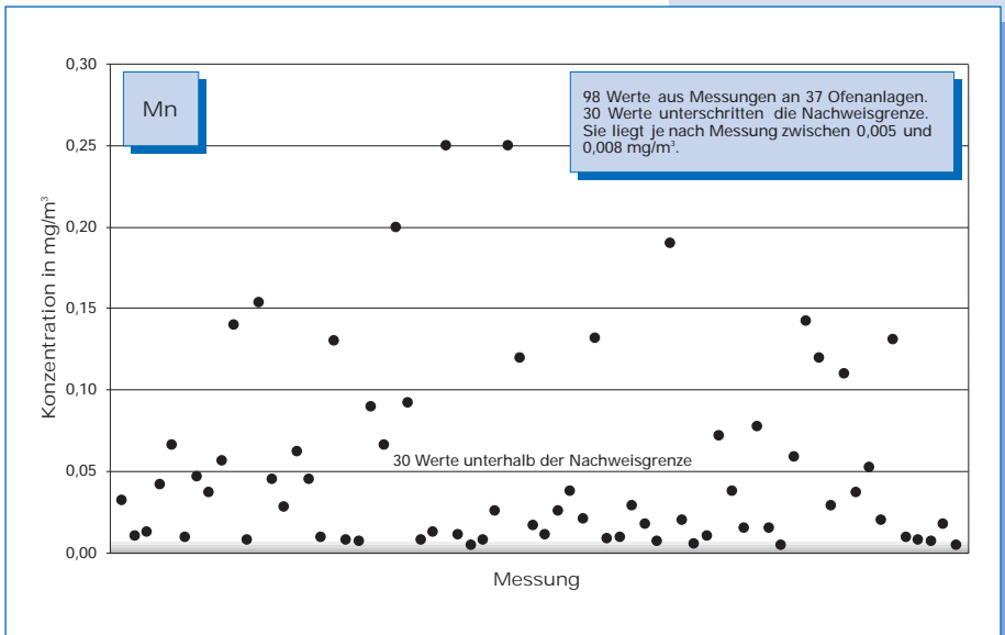
Bild 5-43: Messwerte (Jahr 2000) der Mangan-Konzentration im Reingas von 37 Drehofenanlagen.
