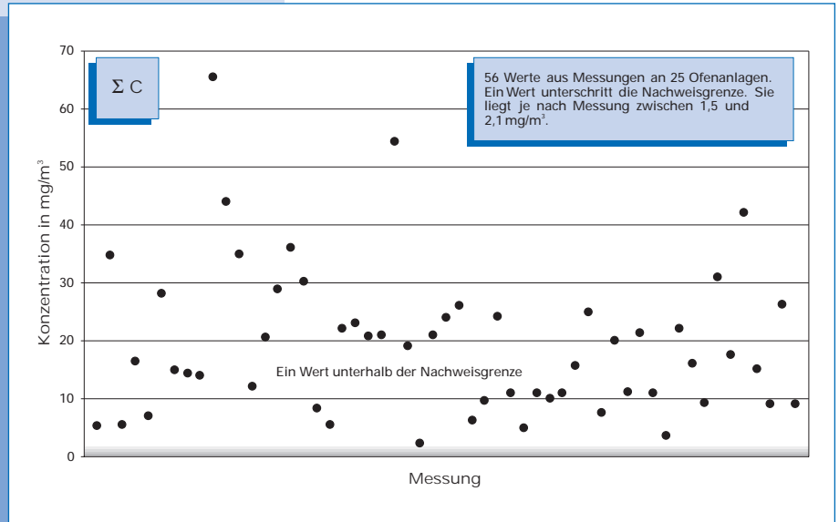
Bild 5-9: Messwerte (Jahr 2000) der Konzentration von organischem Gesamtkohlenstoff im Reingas von 25 Drehofenanlagen.
