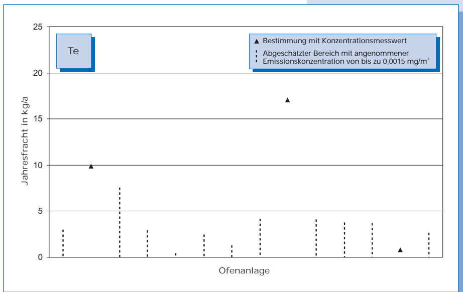
Bild 5-56: Tellur-Emissionen (Jahresfracht 2000) von 14 Drehofenanlagen. Bei Messungen unterhalb der Nachweisgrenze kann die Fracht nur abgeschätzt werden. Der Bereich möglicher Emissionen ist in diesen Fällen als gestrichelte Linie dargestellt, deren Obergrenze mit einer Konzentration von 0,0015 mg/m 3 berechnet wurde.
