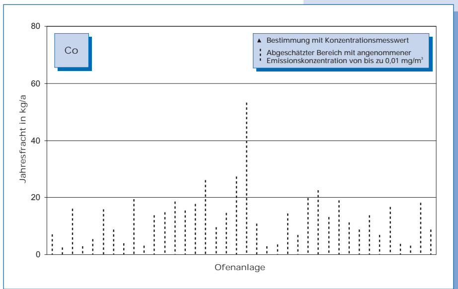
Bild 5-40: Cobalt-Emissionen (Jahresfracht 2000) von 38 Drehofenanlagen.
