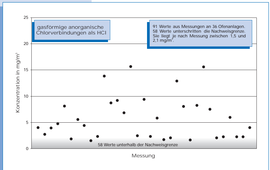
Bild 5-21: Messwerte (Jahr 2000) der Konzentrationen gasförmiger anorganischer Chlorverbindungen, berechnet als HCl, im Reingas von 36 Drehofenanlagen.
