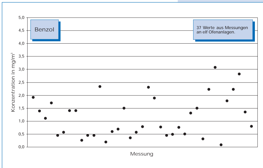
Bild 5-19: Messwerte (Jahr 2000) der Konzentration von Benzol im Reingas von elf Drehofenanlagen.
