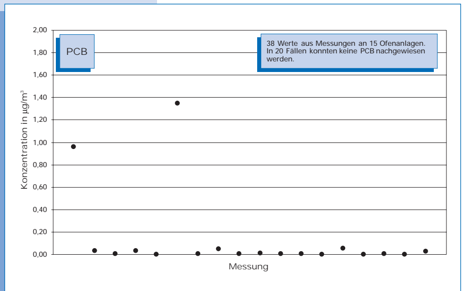
Bild 5-13: Messwerte (Jahr 2000) der Konzentration von polychlorierten Biphenylen (PCB nach DIN 51527) im Reingas von 15 Drehofenanlagen. In 20 Fällen konnten keine PCB nachgewiesen werden. Anmerkung: Für die Messung von PCB im Reingas von Drehofenanlagen gibt es keine genormte Prüfvorschrift, in der Verfahrenskenngrößen des eingesetzten Messverfahrens genannt werden. Deshalb wird hier auf die Angabe einer Nachweisgrenze verzichtet. Bei den derzeit eingesetzten Verfahren sind gemessene Emissionskonzentrationen unterhalb von 0,02 \mu\text{g}/\text{m}^3 nicht abgesichert.
