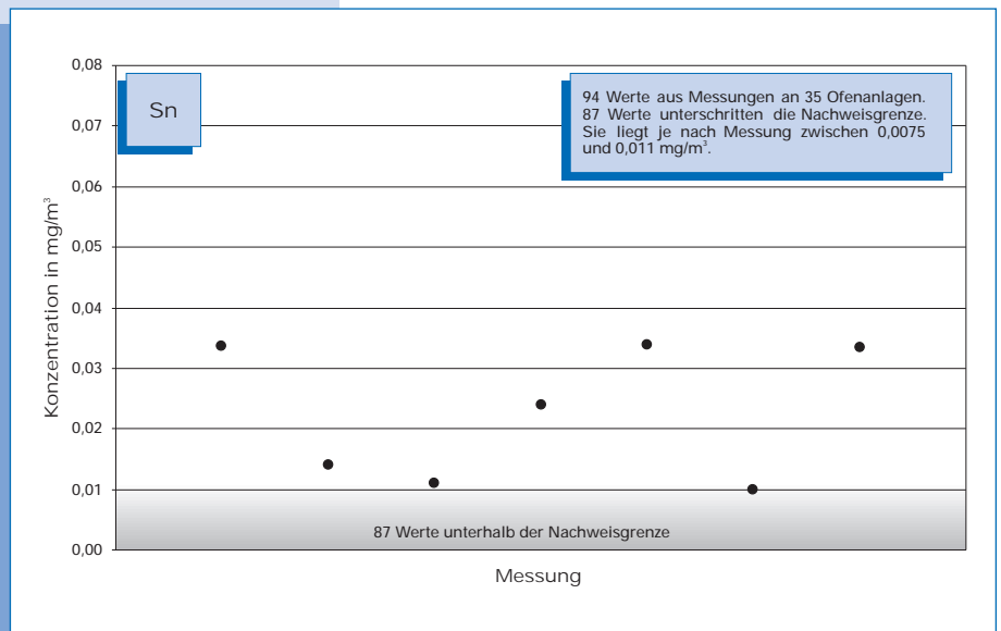
Bild 5-49: Messwerte (Jahr 2000) der Zinn-Konzentration im Reingas von 35 Drehofenanlagen.
