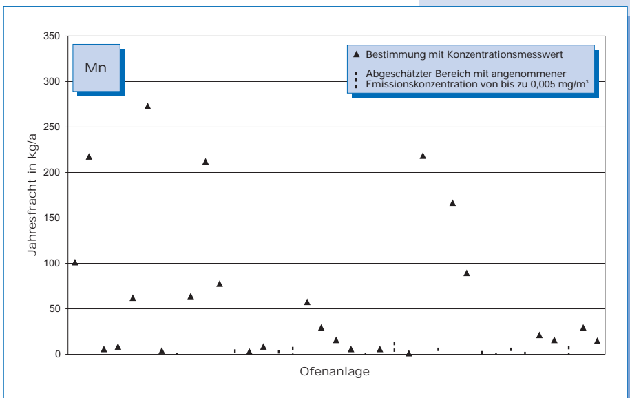
Bild 5-44: Mangan-Emissionen (Jahresfracht 2000) von 37 Drehofenanlagen. Bei Messungen unterhalb der Nachweisgrenze kann die Fracht nur abgeschätzt werden. Der Bereich möglicher Emissionen ist in diesen Fällen als gestrichelte Linie dargestellt, deren Obergrenze mit einer Konzentration von 0,005 mg/m 3 berechnet wurde.
