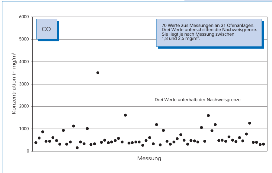
Bild 5-7: Messwerte (Jahr 2000) der CO-Konzentration im Reingas von 31 Drehofenanlagen.
