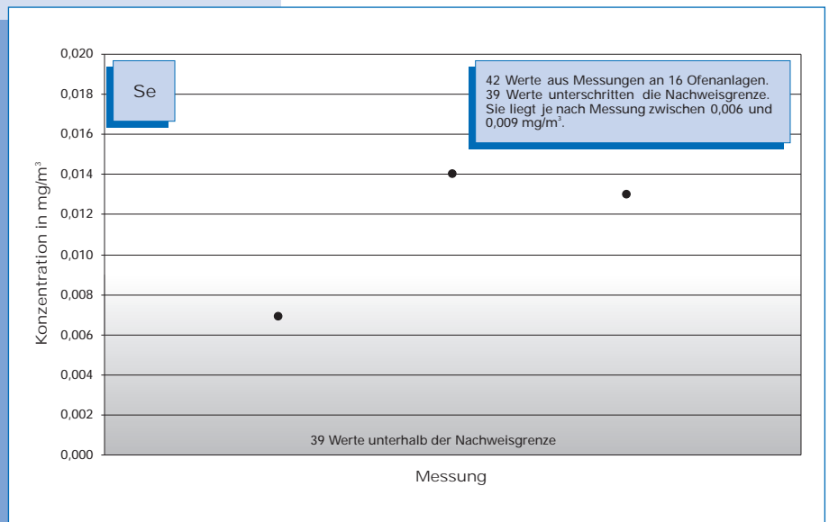
Bild 5-53: Messwerte (Jahr 2000) der Selen-Konzentration im Reingas von 16 Drehofenanlagen.
