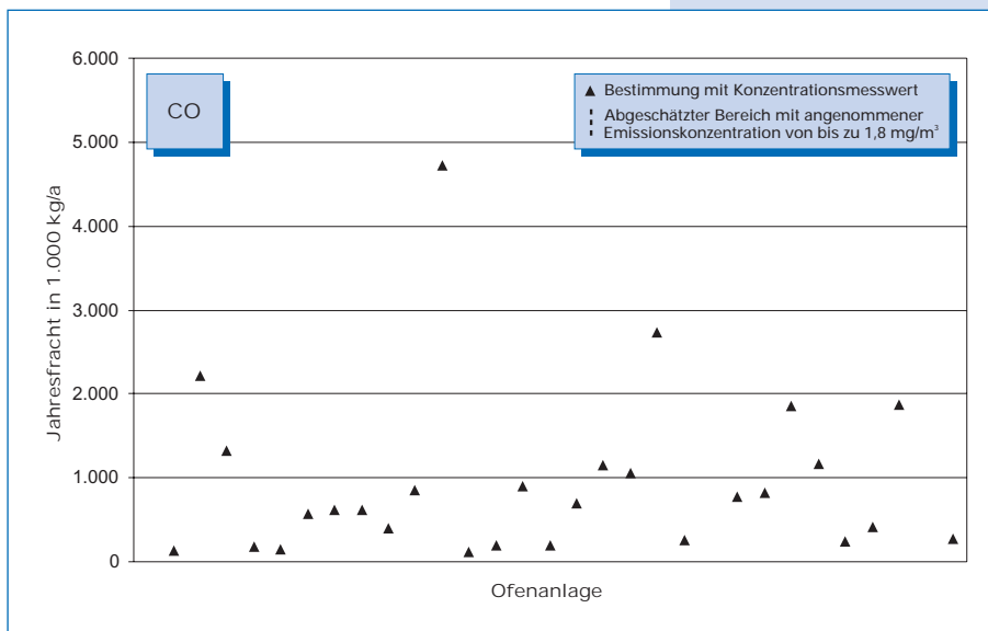
Bild 5-8: CO-Emissionen (Jahresfracht 2000) von 31 Drehofenanlagen. Bei Messungen unterhalb der Nachweisgrenze kann die Fracht nur abgeschätzt werden. Der Bereich möglicher Emissionen ist in diesen Fällen als gestrichelte Linie dargestellt, deren Obergrenze mit einer Konzentration von 1,8 mg/m 3 berechnet wurde.
