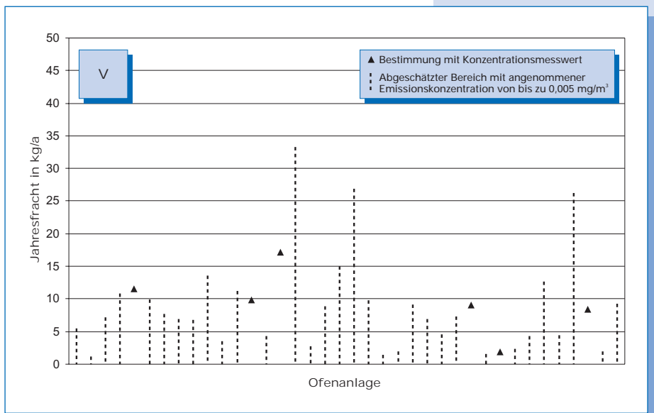
Bild 5-48: Vanadium-Emissionen (Jahresfracht 2000) von 38 Drehofenanlagen. Bei Messungen unterhalb der Nachweisgrenze kann die Fracht nur abgeschätzt werden. Der Bereich möglicher Emissionen ist in diesen Fällen als gestrichelte Linie dargestellt, deren Obergrenze mit einer Konzentration von 0,005 mg/m 3 berechnet wurde.
