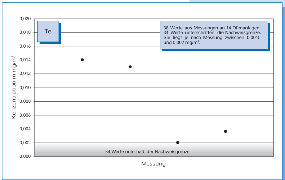
Bild 5-55: Messwerte (Jahr 2000) der Tellur-Konzentration im Reingas von 14 Drehofenanlagen.
