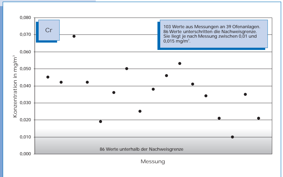
Bild 5-37: Messwerte (Jahr 2000) der Chrom-Konzentration im Reingas von 39 Drehofenanlagen.
