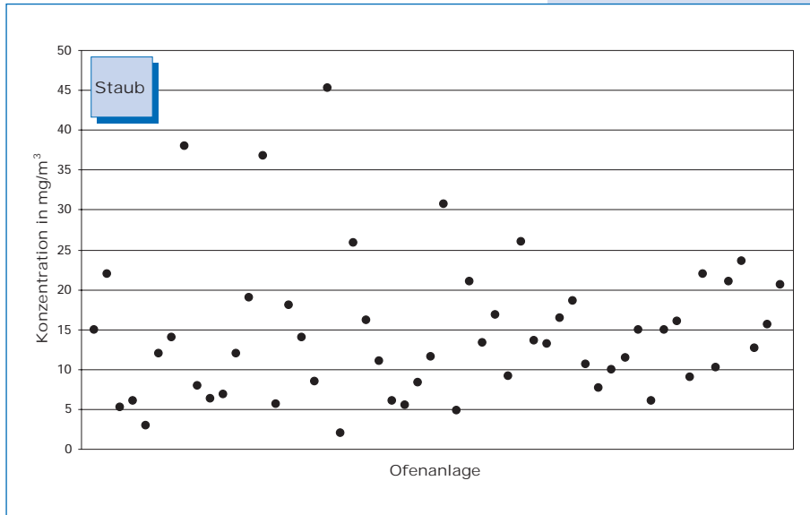
Bild 5-1: Mittelwerte (Jahr 2000) der Staubkonzentration im Reingas von 54 Drehofenanlagen.
