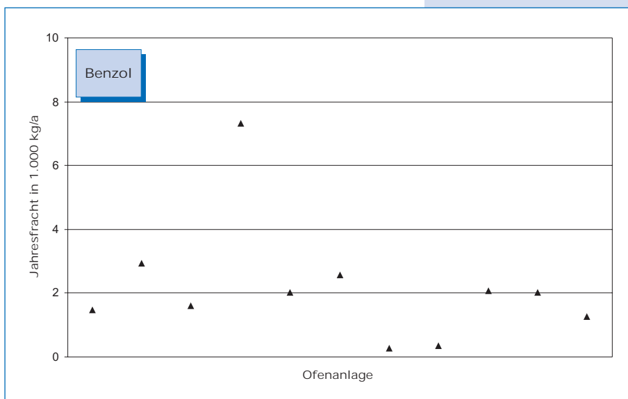
Bild 5-20: Benzol-Emissionen (Jahresfracht 2000) von elf Drehofenanlagen.
