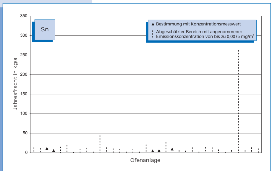
Bild 5-50: Zinn-Emissionen (Jahresfracht 2000) von 35 Drehofenanlagen. Bei Messungen unterhalb der Nachweisgrenze kann die Fracht nur abgeschätzt werden. Der Bereich möglicher Emissionen ist in diesen Fällen als gestrichelte Linie dargestellt, deren Obergrenze mit einer Konzentration von 0,0075 mg/m 3 berechnet wurde.
