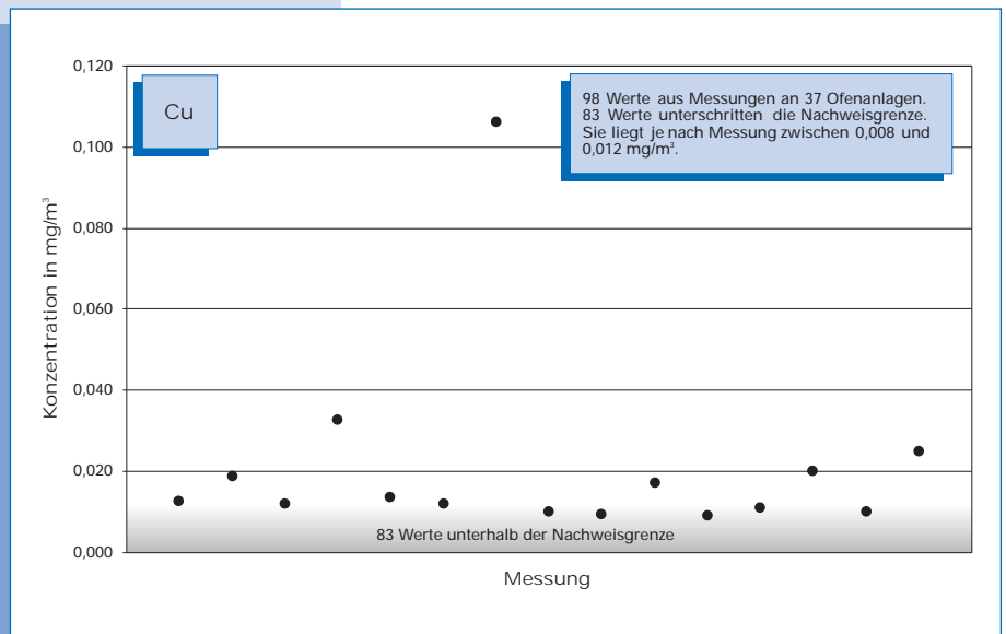
Bild 5-41: Messwerte (Jahr 2000) der Kupfer-Konzentration im Reingas von 37 Drehofenanlagen.
