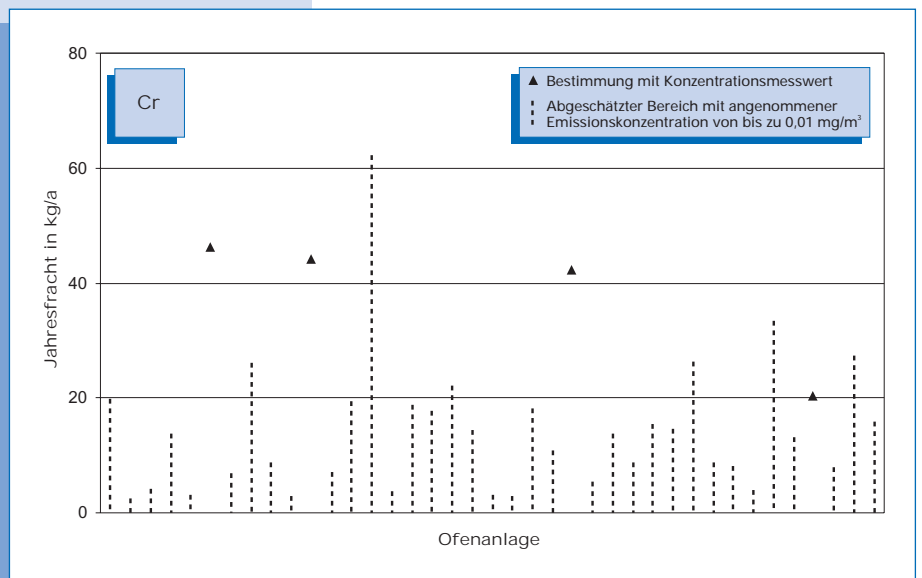
Bild 5-38: Chrom-Emissionen (Jahresfracht 2000) von 39 Drehofenanlagen. Bei Messungen unterhalb der Nachweisgrenze kann die Fracht nur abgeschätzt werden. Der Bereich möglicher Emissionen ist in diesen Fällen als gestrichelte Linie dargestellt, deren Obergrenze mit einer Konzentration von 0,01 mg/m 3 berechnet wurde.
