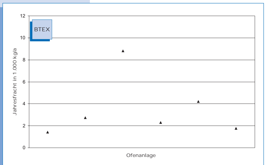
Bild 5-18: BTEX-Emissionen (Jahresfracht 2000) von sechs Drehofenanlagen.
