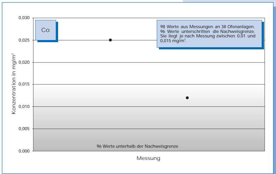
Bild 5-39: Messwerte (Jahr 2000) der Cobalt-Konzentration im Reingas von 38 Drehofenanlagen.
