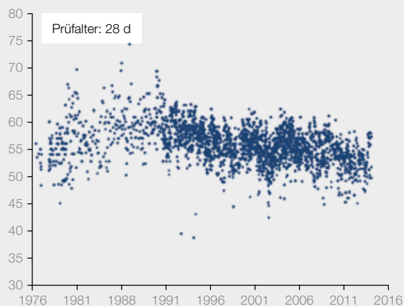
Abbildung 6.4: Druckfestigkeit von Normmörteln eines Referenzzements (CEM I 42,5 R) im Alter von 28 Tagen (Quelle: ibac RWTH Aachen)
